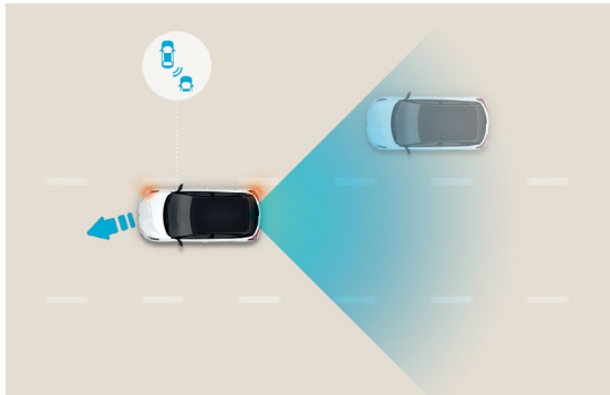
מערכת אקטיבית לזיהוי ומניעת התנגשות בעת מעבר נתיב (BCA)* מערכת מבוססת רדאר המתריעה על רכבים ב"שטח מת" ומבצעת תיקון אקטיבי בעת מעבר לנתיב שאינו פנוי.
